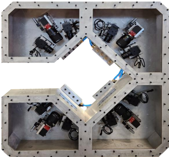
센서하우징 (내부 센서는 별도)
